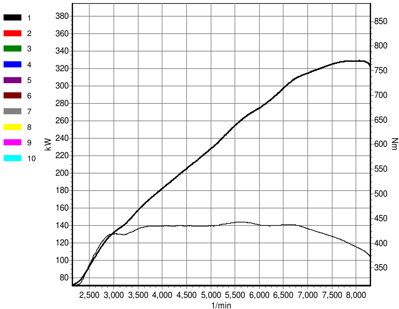
P-max Motorleistung (korr.) / Geschwindigkeit / Drehmoment (korr.)
